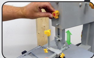
Guide lames réglable en hauteur Adjustable blade guide
