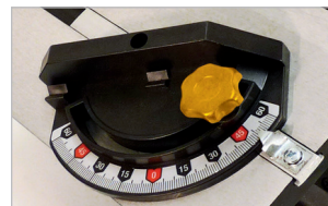
Guide d'onglet Mitre guide
